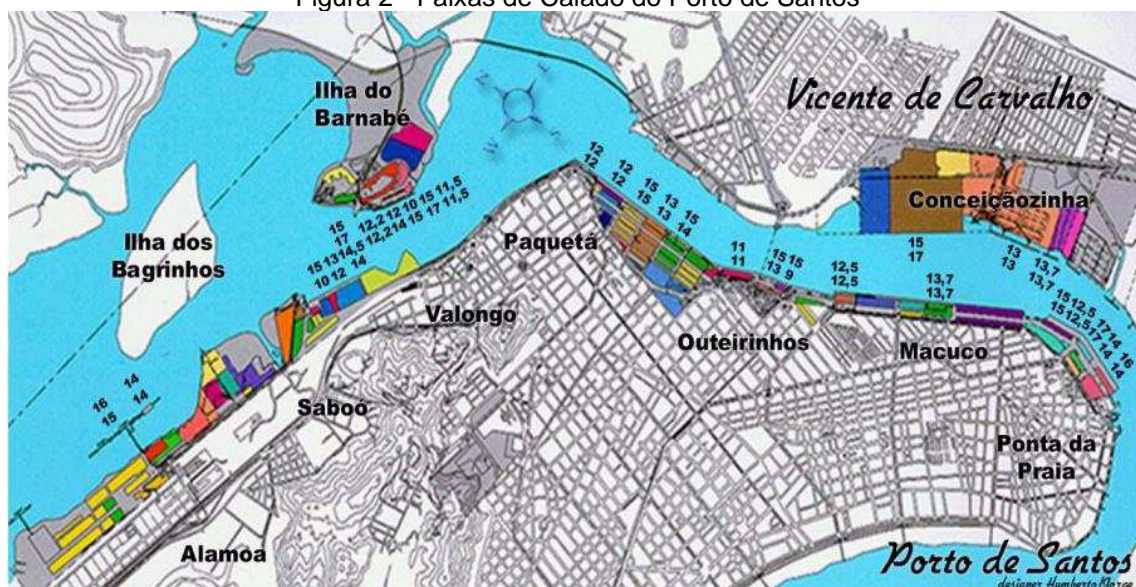
Figura 2 - Faixas de Calado do Porto de Santos
